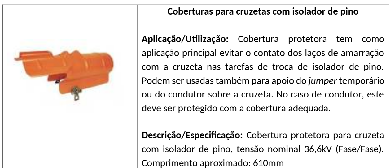
Figura 109 - Coberturas para cruzetas com isolador de pino
