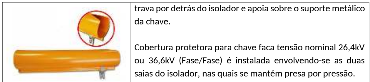
Figura 107 - Coberturas para chaves faca e fusível
