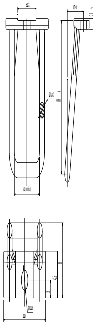
Figura 73 - Estribo para braço tipo L
