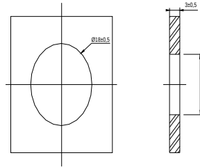
Figura 14 - Arruela quadrada
