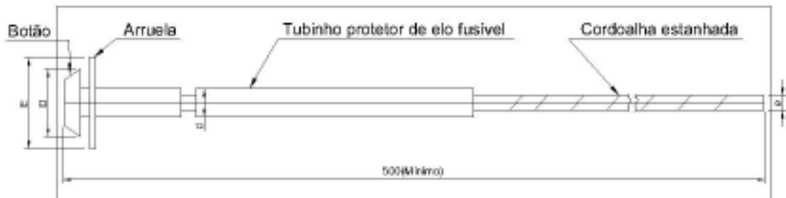
Figura 67 - Elo fusível
