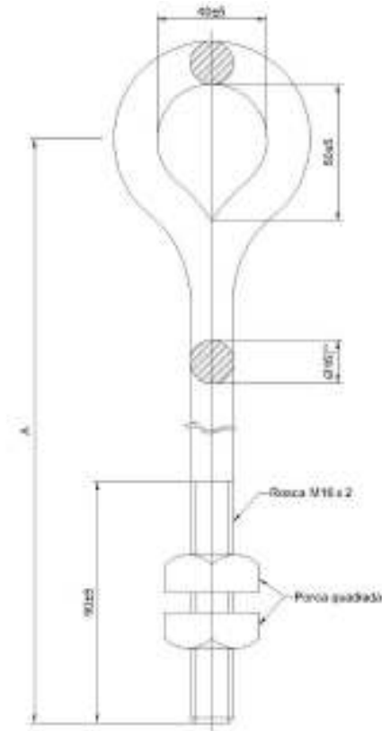
Figura 82 - haste de âncora para estai
