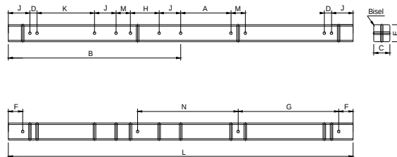
Figura 57 - Cruzeta de concreto armado de 2400mm
