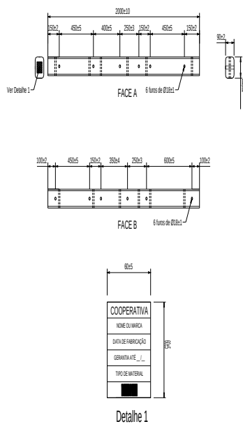
Figura 65 - Cruzeta em fibra de vidro de seção retangular 2000mm
