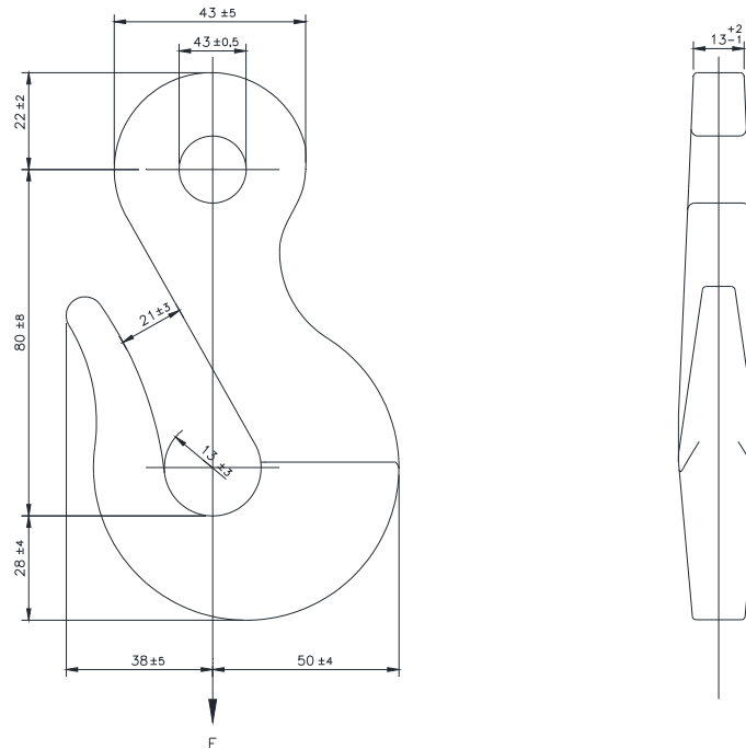
Figura 78 - Gancho olhal
