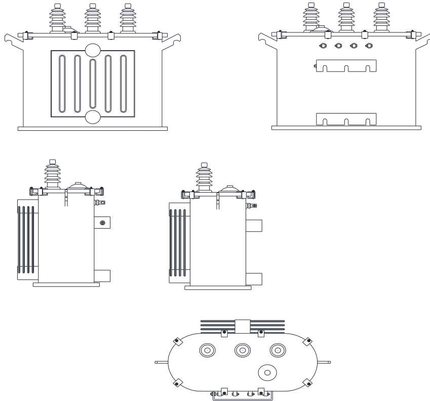
Figura 137 - Transformador abaixador de tensão trifásico
