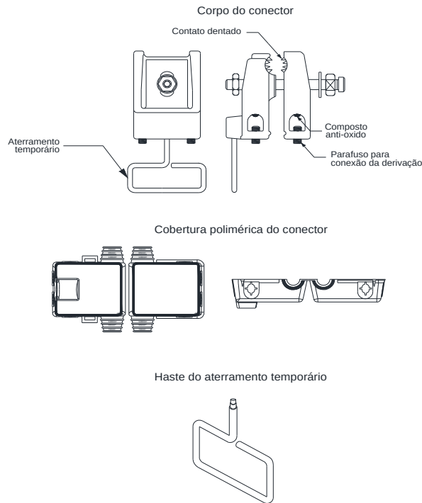
Figura 47 - Conector multiderivações com estribo
