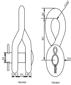
Figura 99 - Manilha torcida
