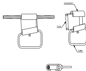
Figura 40 - Conector de cunha com estribo
