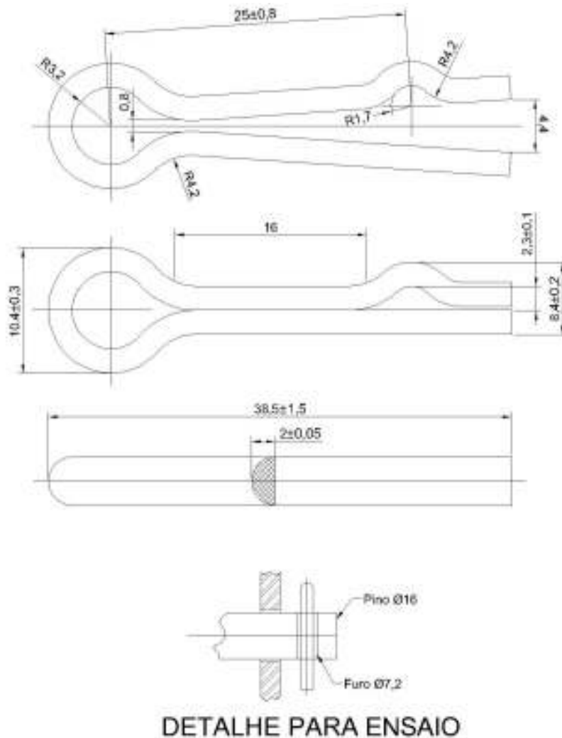
Figura 66 - Cupilha
