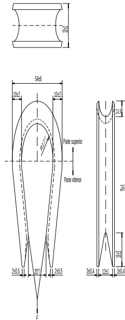
Figura 121 - Sapatilha
