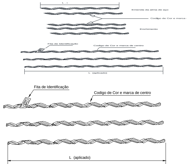
Figura 69 - Emenda pré-formada total para cabo CAA
