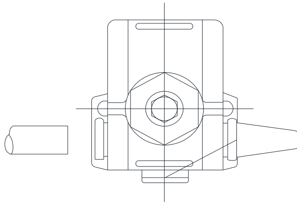
Figura 44 - Conector de perfuração
