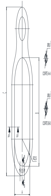
Figura 10 - Anel de amarração para isolador polimérico e espaçadores losangulares
