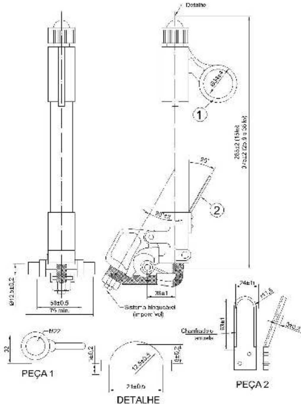
Figura 28 - Cartucho para chave fusível
