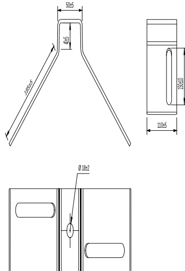
Figura 125 - Suporte afastador vértice
