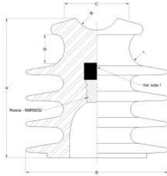
Figura 88 - Isolador polimérico tipo pino
