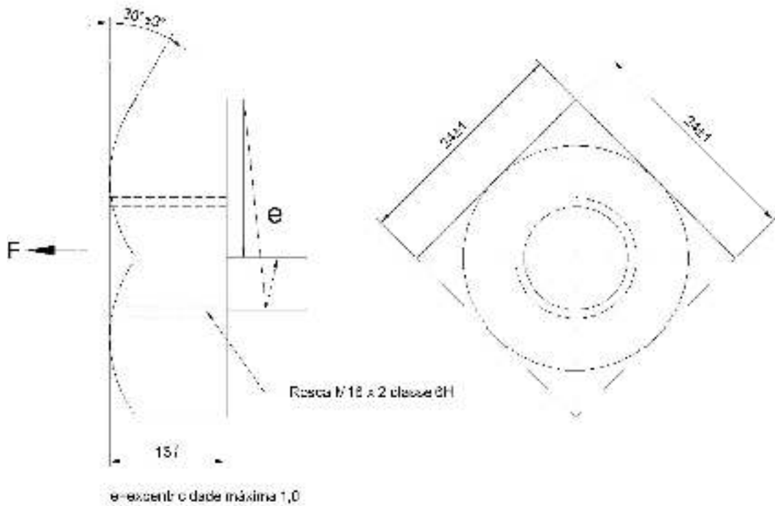
Figura 115 - Porca quadrada
