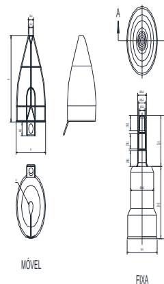
Figura 27 - Capa protetora polimérica para bucha ou para-raios
