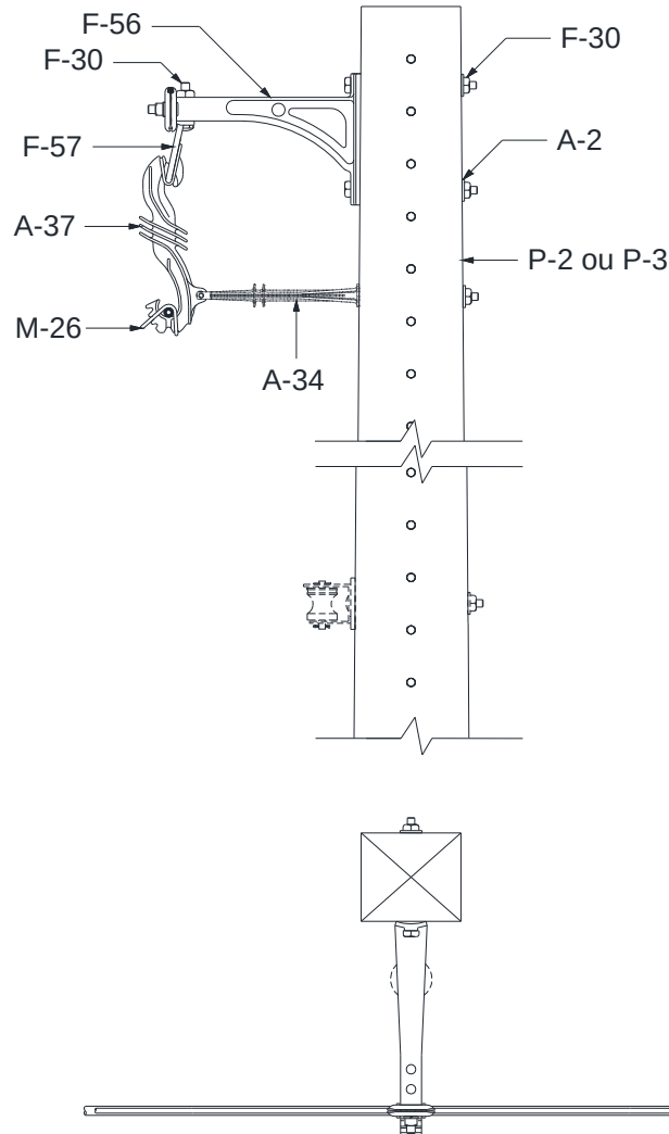
Figura 21 - Estrutura CU1A - Poste de concreto de seção DT ou de madeira
