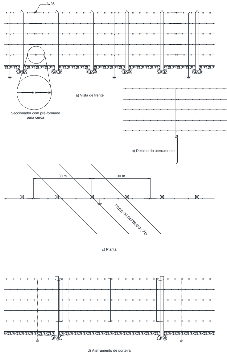
Figura 101 – Seccionamento de cerca – Cerca paralela
