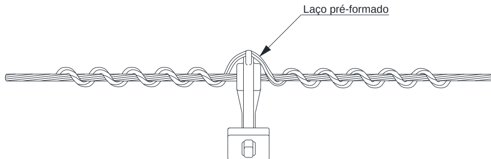
Figura 86 - Amarrações e ligações - Amarração do espaçador monofásico, vertical e losangular em cordoalha - Laço pré-formado
