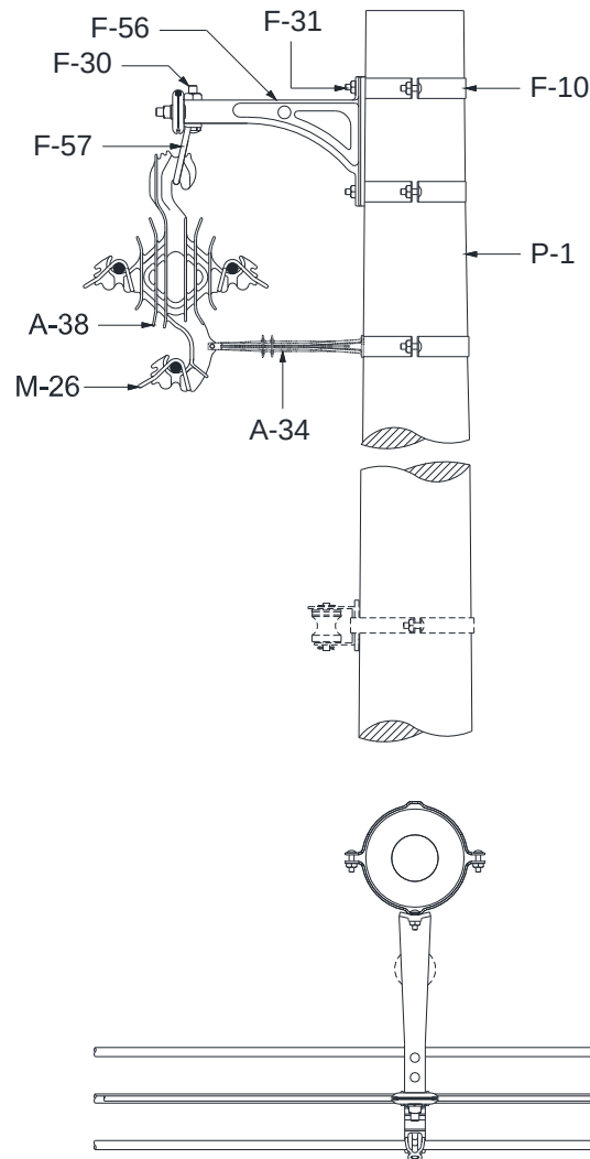
Figura 28 - Estrutura CA1 - Poste de concreto de seção circular
