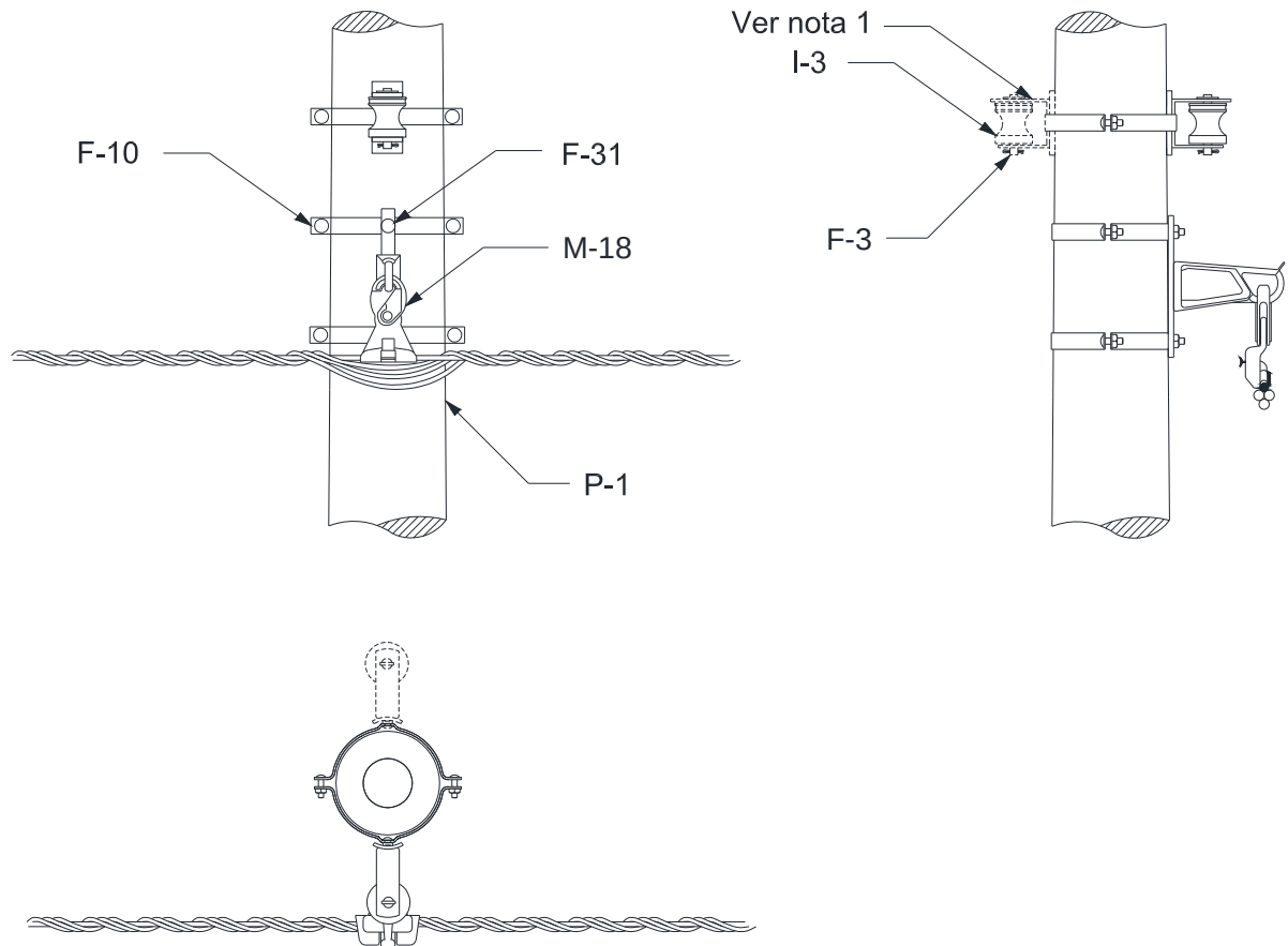
Figura 10 – Estruturas tangentes – SI1 – Poste de concreto de seção circular
