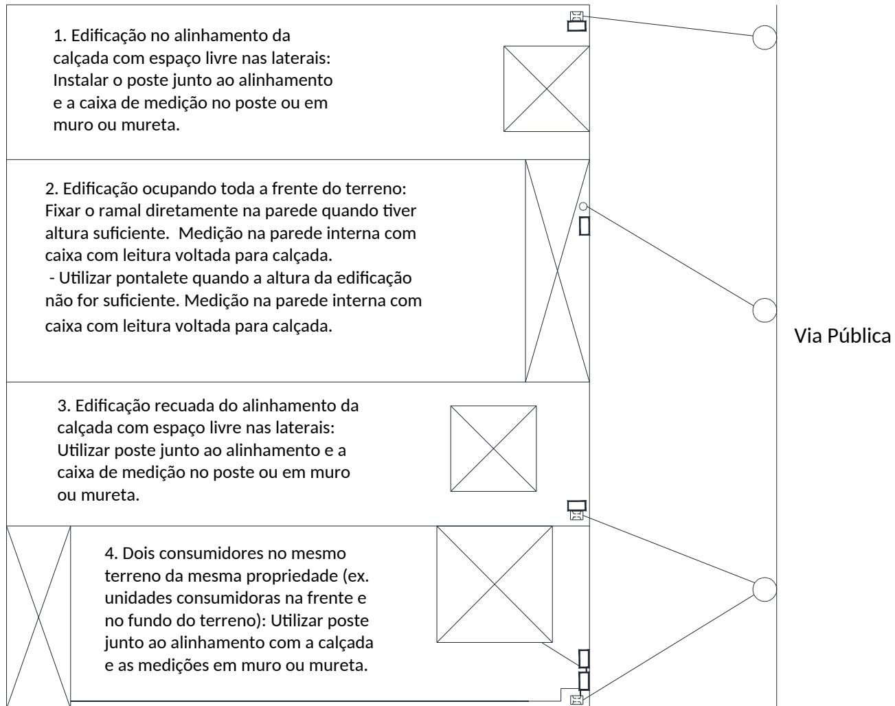
Figura 1 - Condições gerais para ramal de ligação
