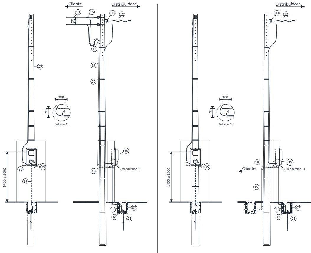
Figura 26 - Padrão de entrada com caixa de medição monofásico em muro - Uma caixa (Rio de Janeiro)
