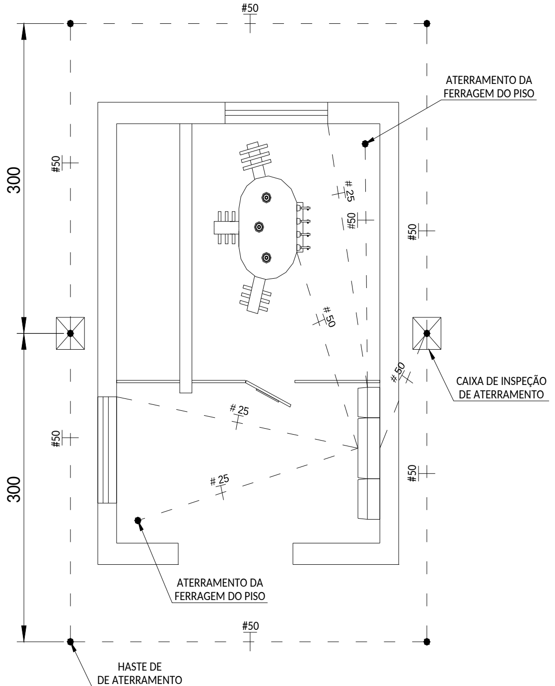
Figura 25 - Esquema típico de eletrodo de aterramento para cabine primária
