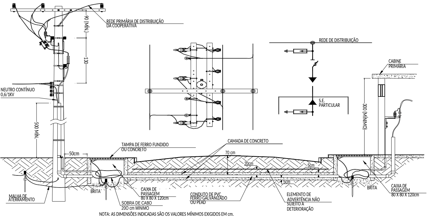
Figura 9 - Ramal de entrada subterrâneo
