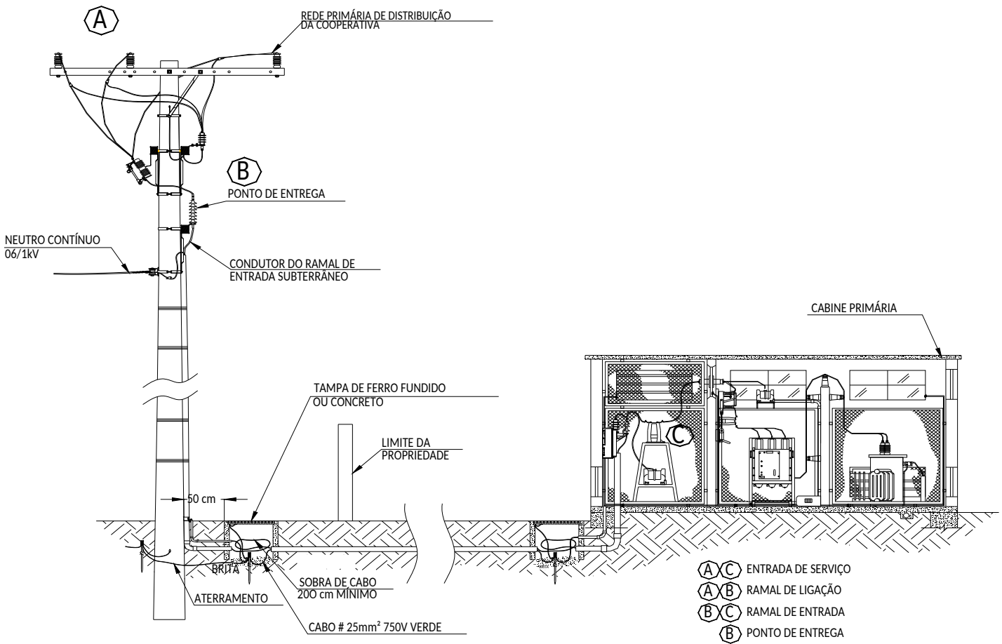
Figura 7 - Elementos componentes da entrada
